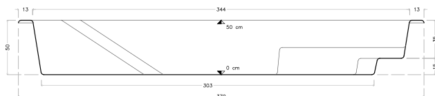
Sección Longitudinal
