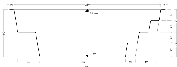
Sección Longitudinal
