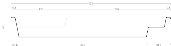
Sección B
