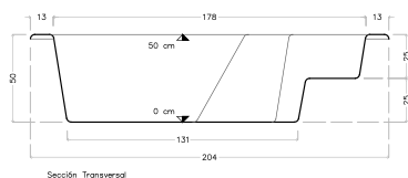
Sección Transversal
