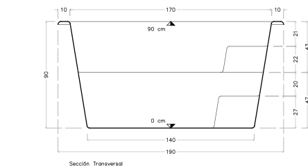
Sección Transversal
